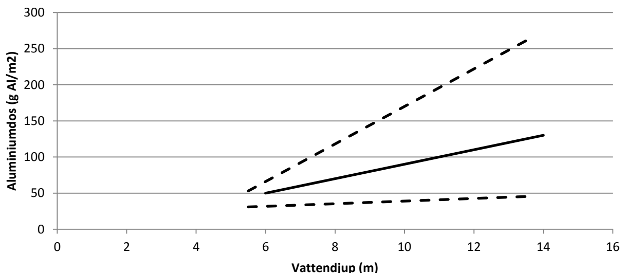
Figur 26. Aluminiumdos som krävs för att binda fosfor i fraktionen Löst bunden fosfor (domineras av fosfat i porvattnet) samt för att binda hela förrådet av läckagebenägen fosfor till 0,5 m sedimentdjup indikeras av nedre respektive övre streckade linjen. Heldragen linje beskriver föreslagen aluminiumdos för olika vattendjup.
