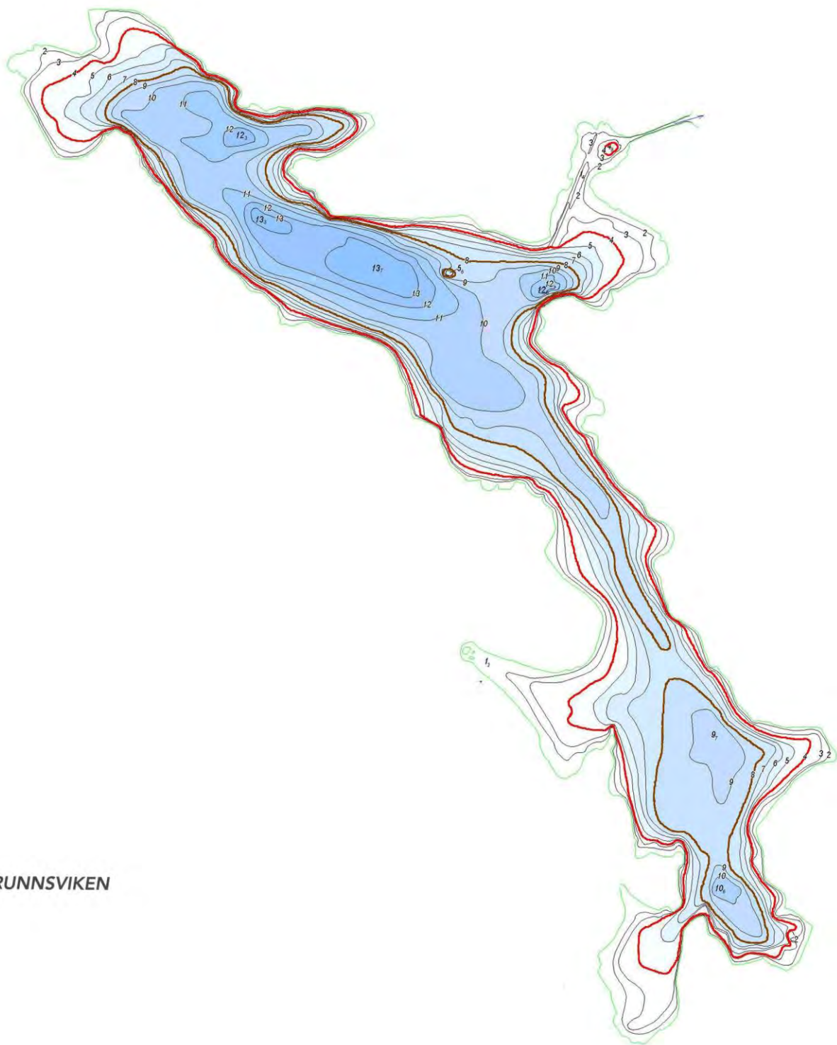
Figur 10. Översiktlig bottendynamisk karta för Brunnsviken baserad på Myricas djupkarta. Gränsen mellan erosions- och transportbottnar (E/T) å ena sidan och ackumulationsbottnar (A) å den andra indikeras med röd linje (4 meters djup). Gränsen mellan oxiderade och reducerade bottnar indikeras av brun linje (8 meters djup).
