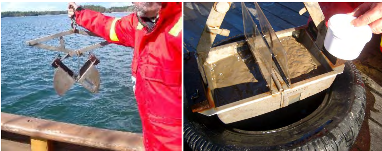
Figur 6 och 7. Vänstra bilden: Ponarhämtaren laddad och redo för hugg. Högra bilden: Ponaren öppnad och klar för ytsedimentprovtagning.
