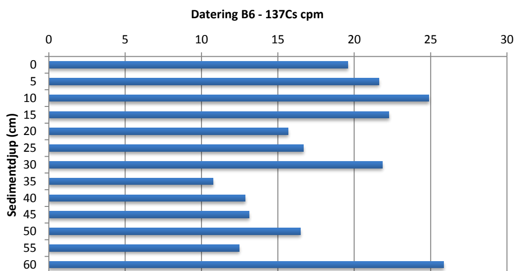
Figur 11. Resultat av dateringsförsök med radiocesium ( ^{137}\text{Cs} ) uttryckt som CPM (Counts Per Minute).
