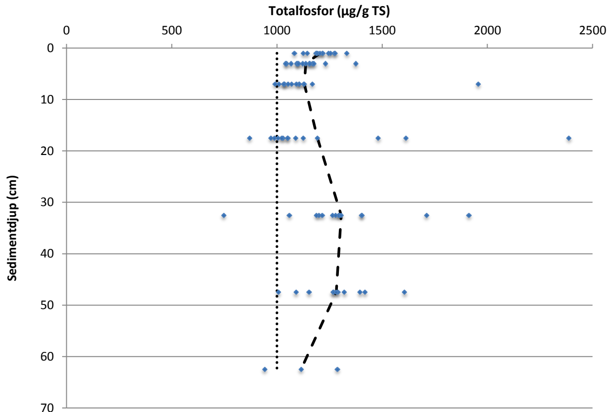
Figur 23. Uppmätta totalhalter av fosfor i Brunnsvikens botten samt antagen begravningskoncentration (1 mg P/g TS).
