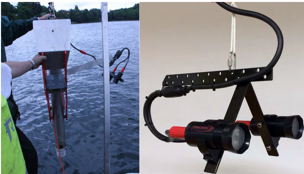
Figur 4 och 5. Geminihämtare med bottenvideokamera monterad på sidoarm för filmning av provtagning vid sedimentytan. Höger bild: Bottenvideokamera Sublight Technology.
